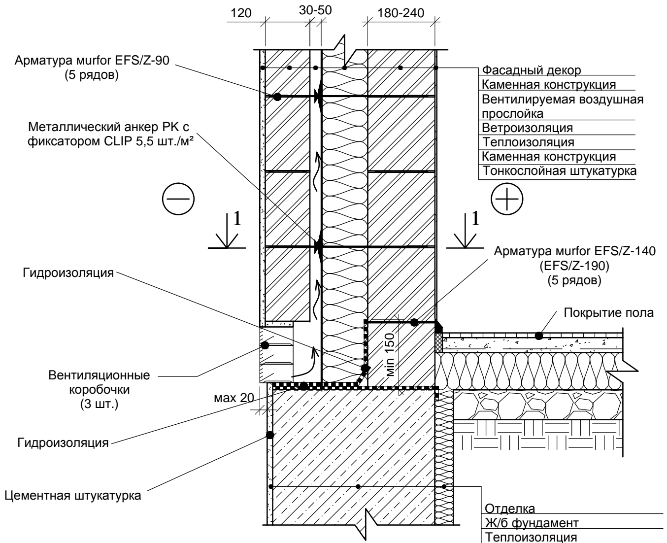
РАЗРЕЗ 1-1
