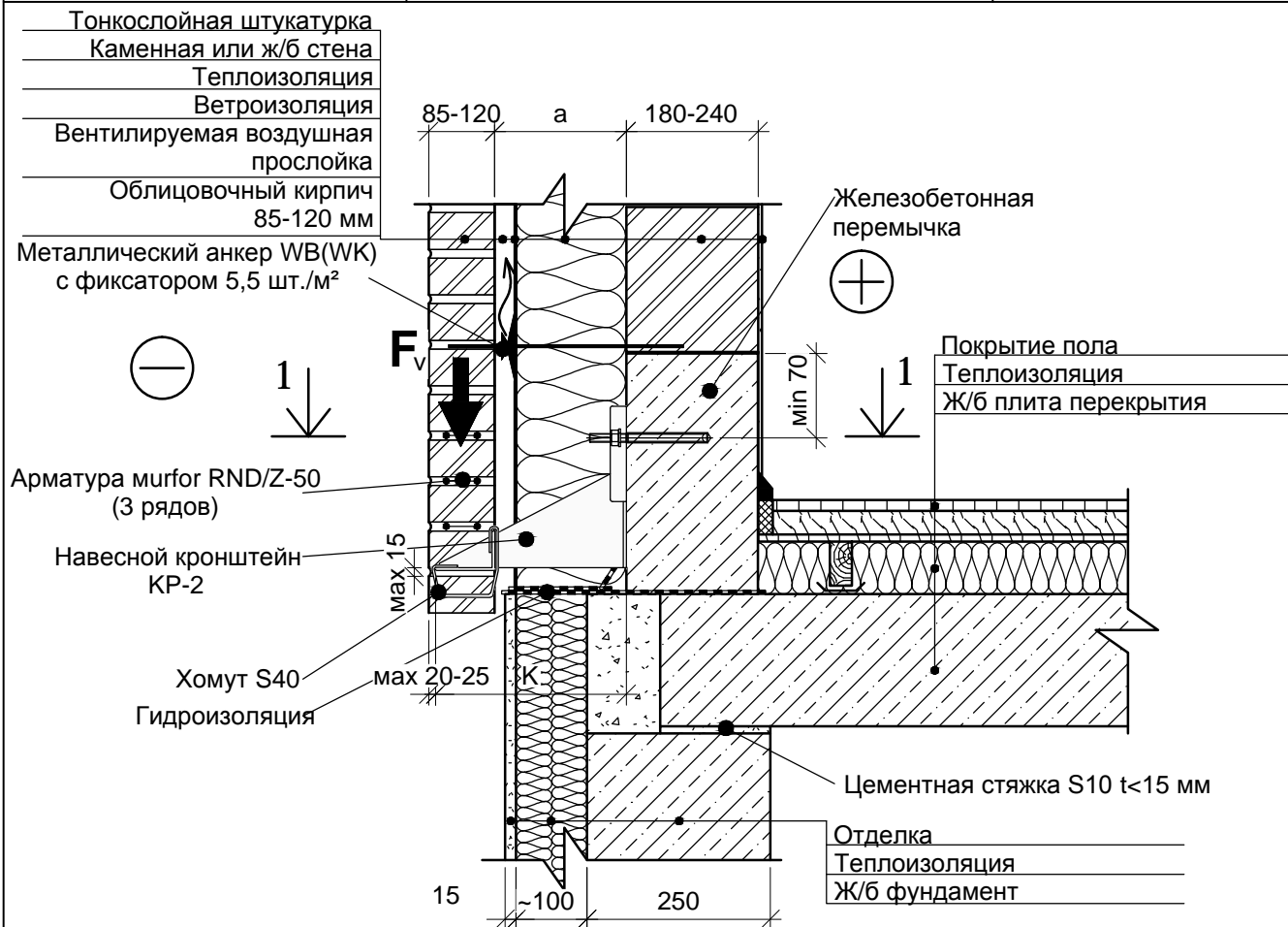
РАЗРЕЗ 1-1
