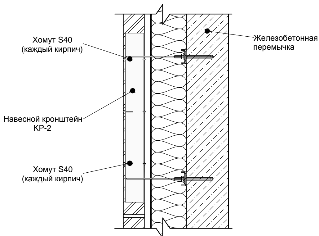
РАЗРЕЗ 1-1
