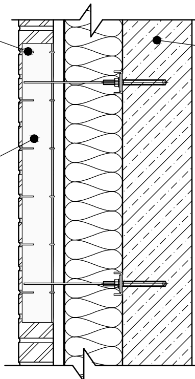
РАЗРЕЗ 1-1
