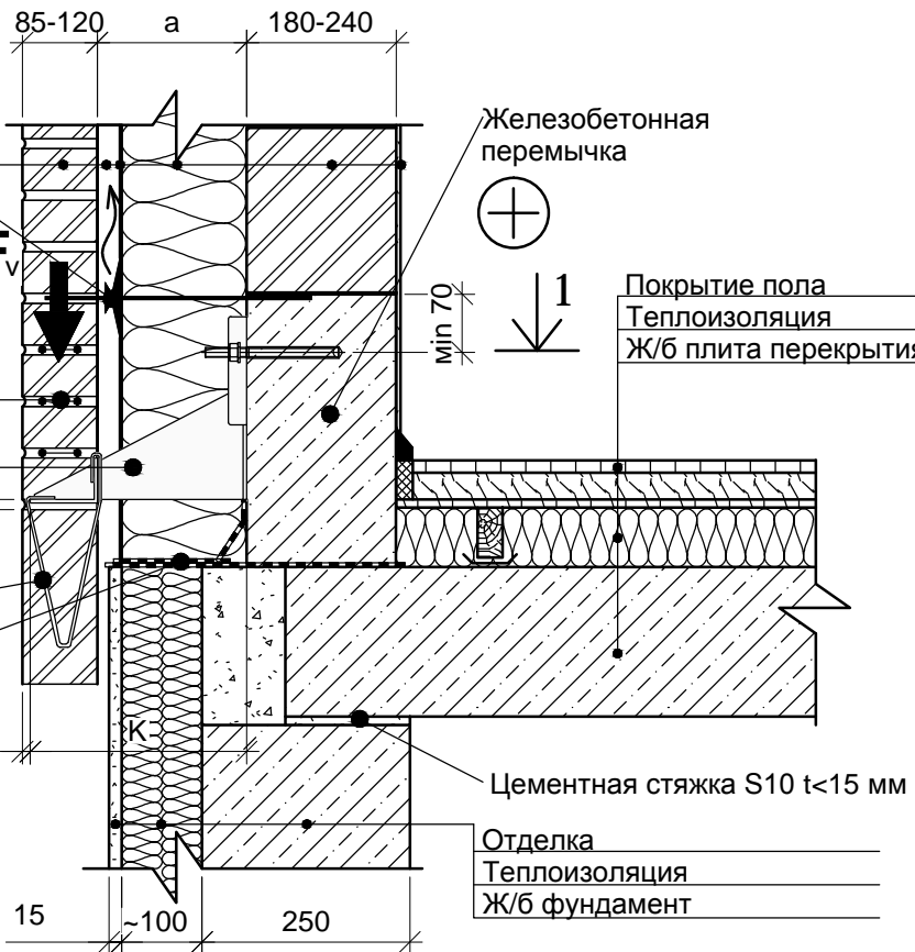
РАЗРЕЗ 1-1
