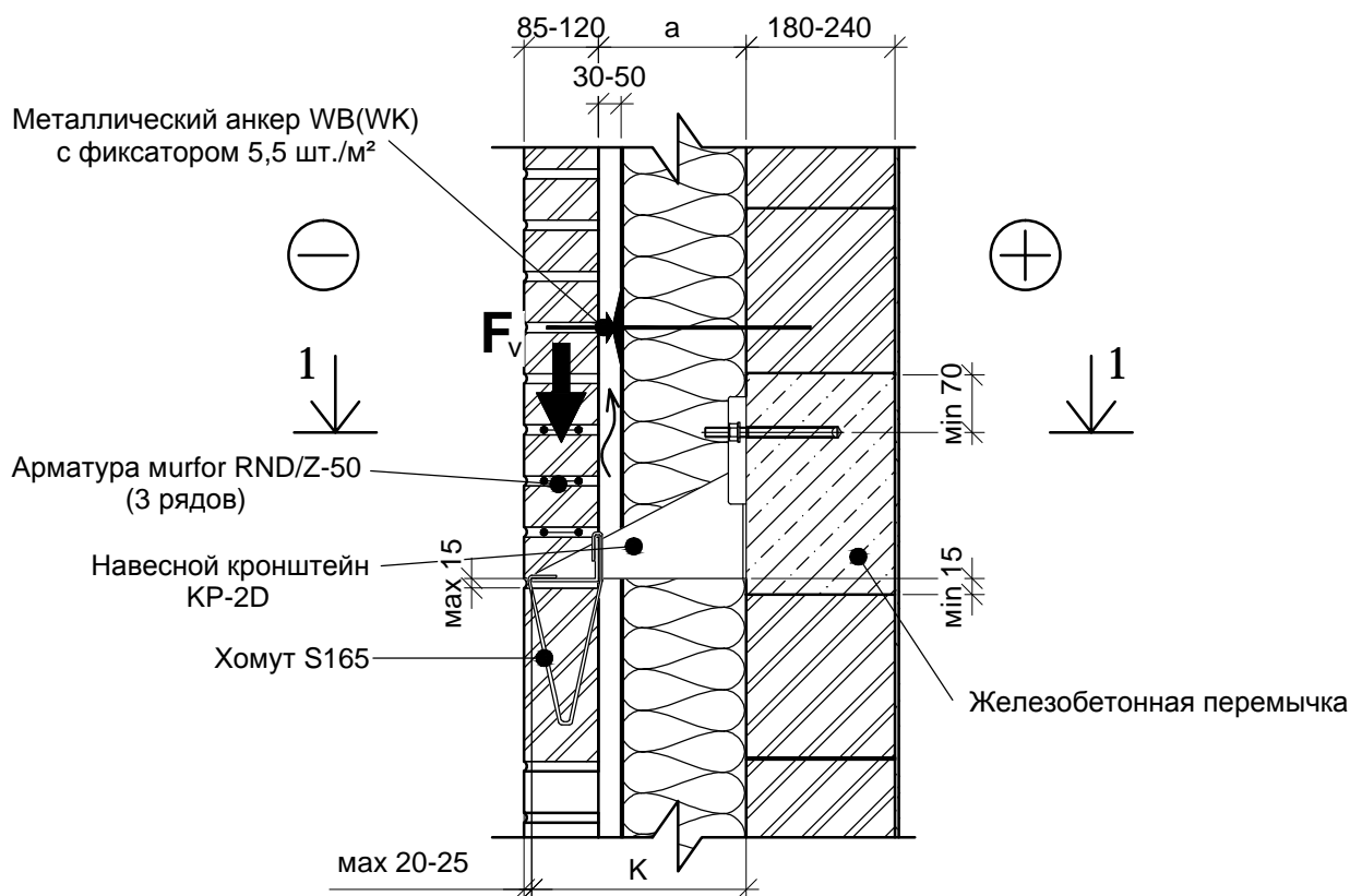
РАЗРЕЗ 1-1
