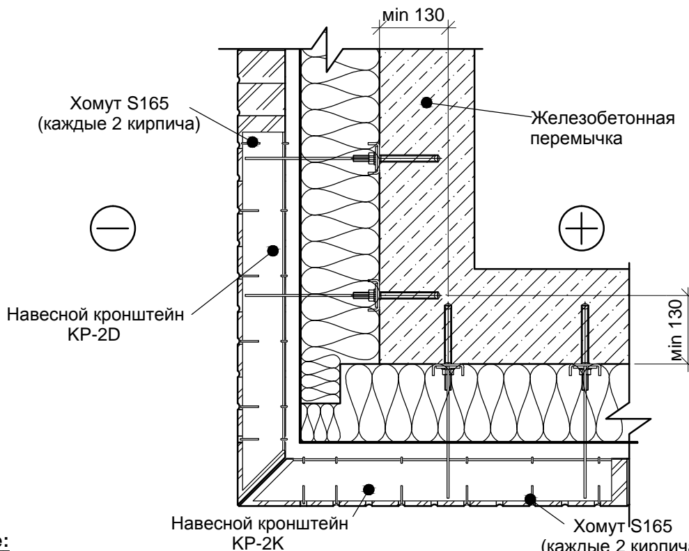
РАЗРЕЗ 1-1
