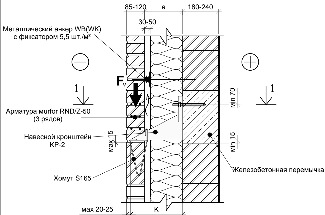
РАЗРЕЗ 1-1
