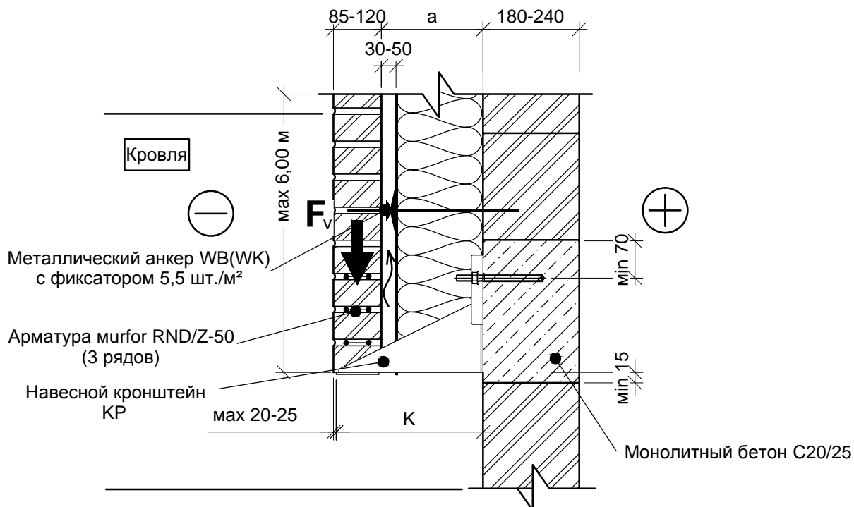
РАЗРЕЗ 1-1
