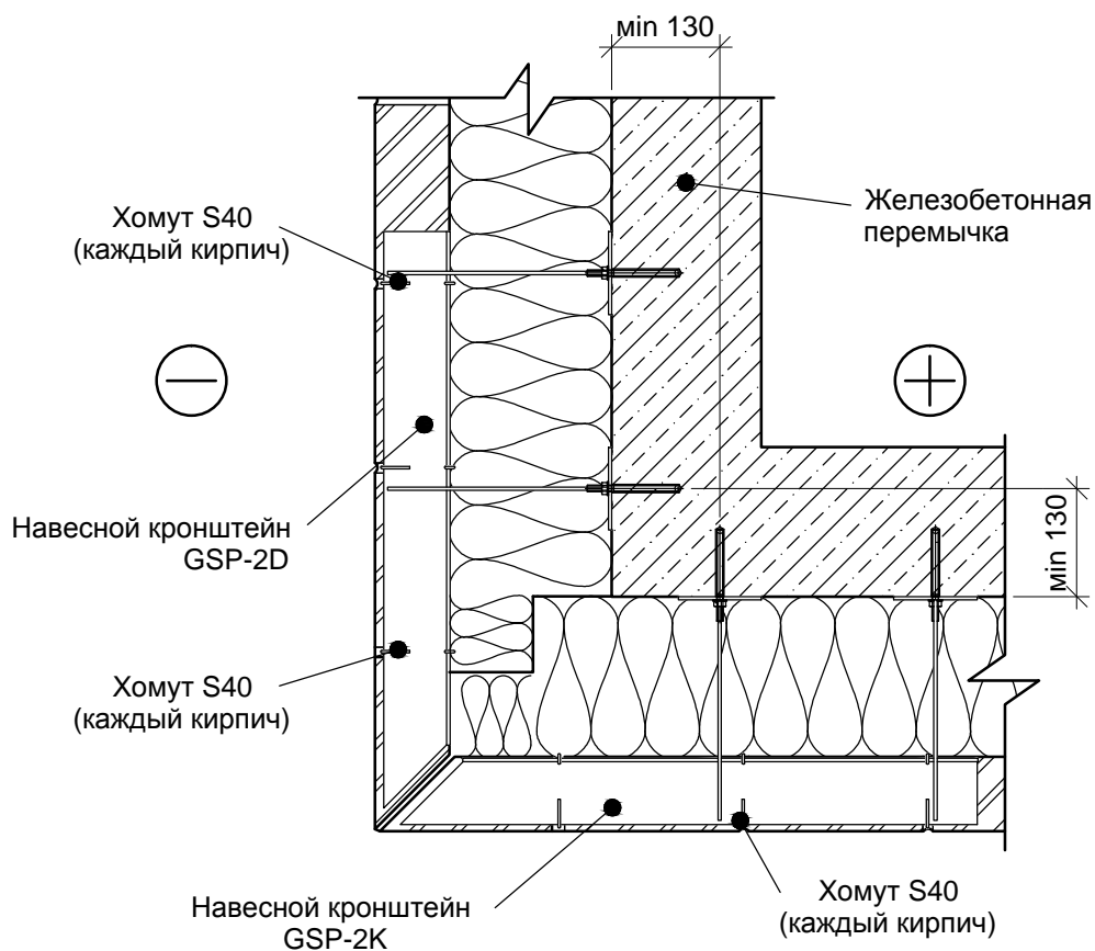
РАЗРЕЗ 1-1
