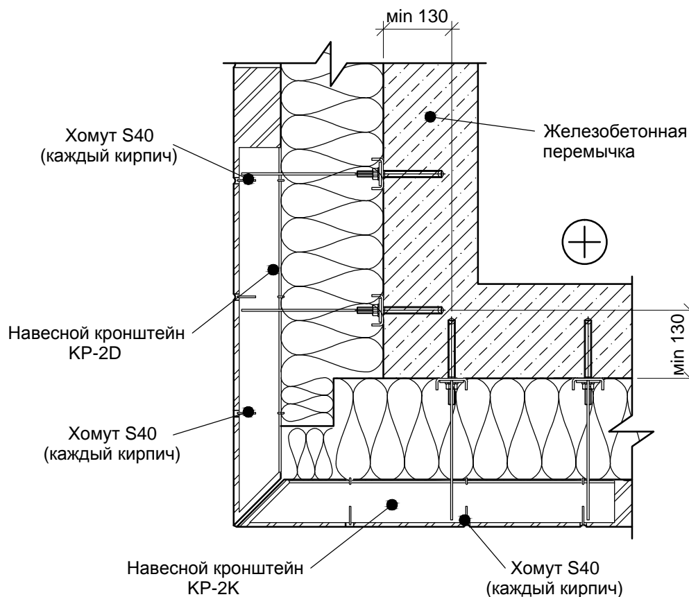
РАЗРЕЗ 1-1
