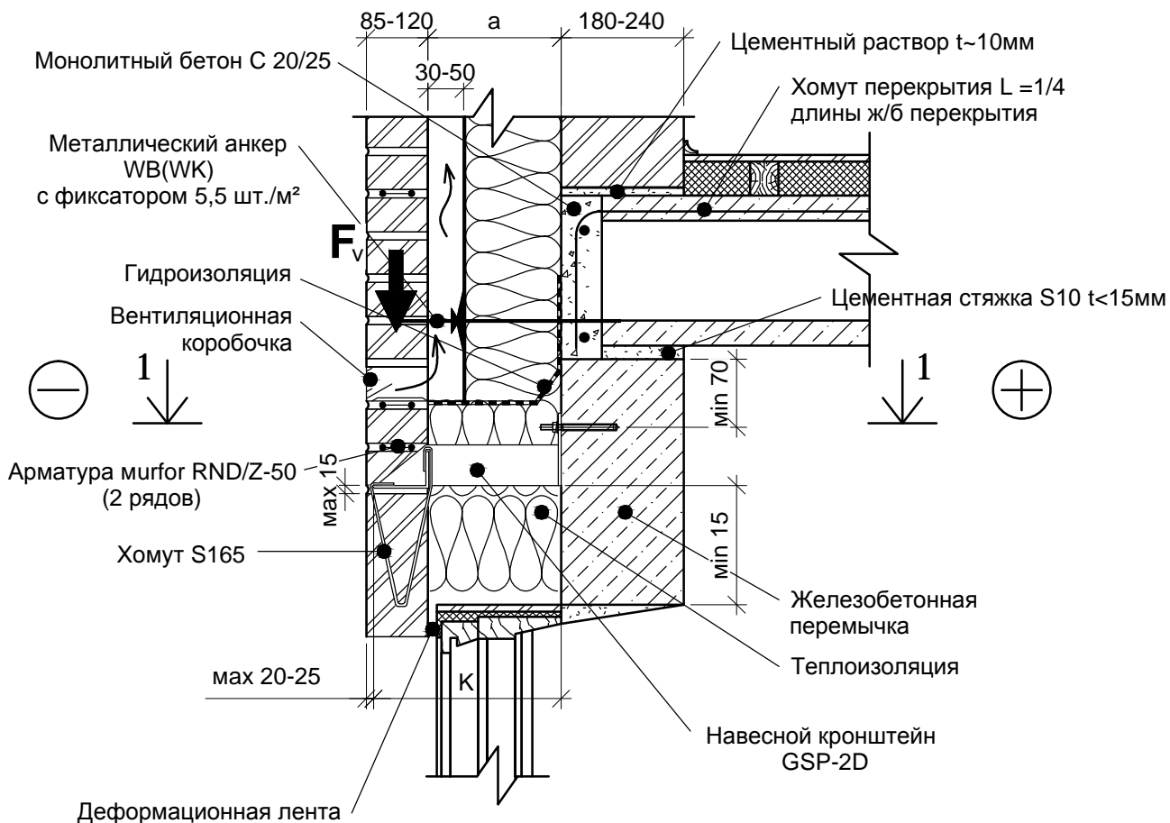
РАЗРЕЗ 1-1
