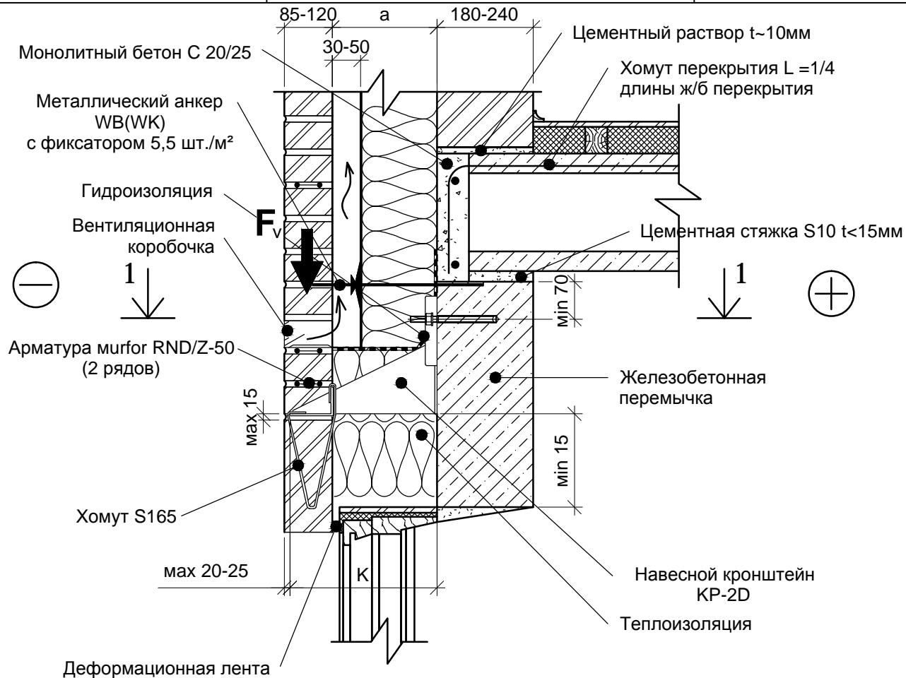
РАЗРЕЗ 1-1
