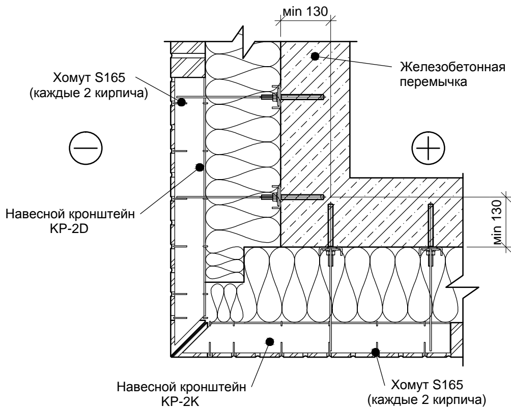
РАЗРЕЗ 1-1
