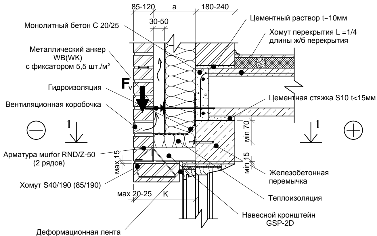
РАЗРЕЗ 1-1
