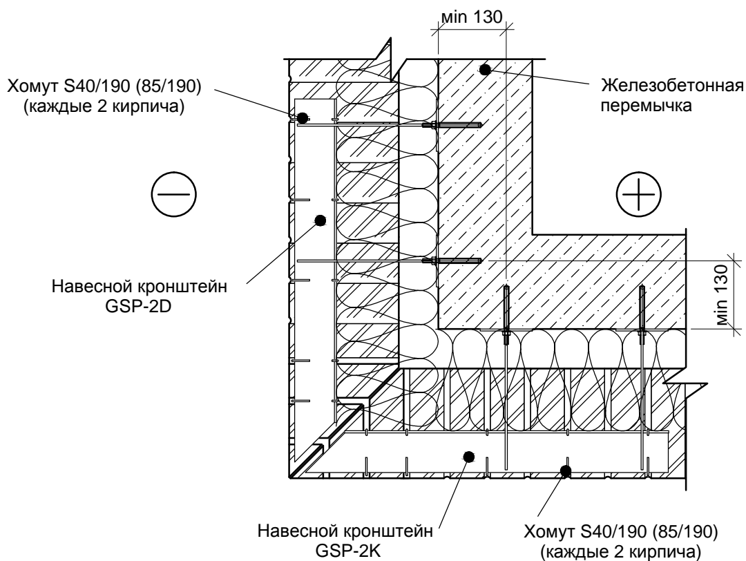
РАЗРЕЗ 1-1
