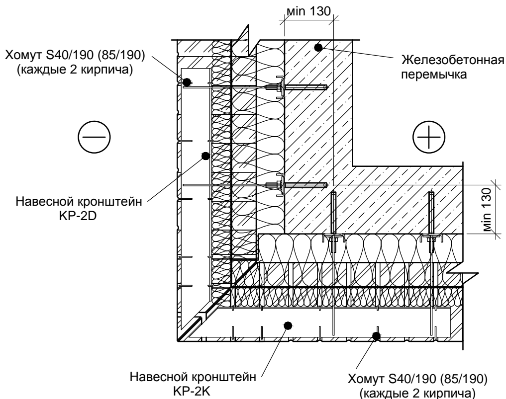
РАЗРЕЗ 1-1
