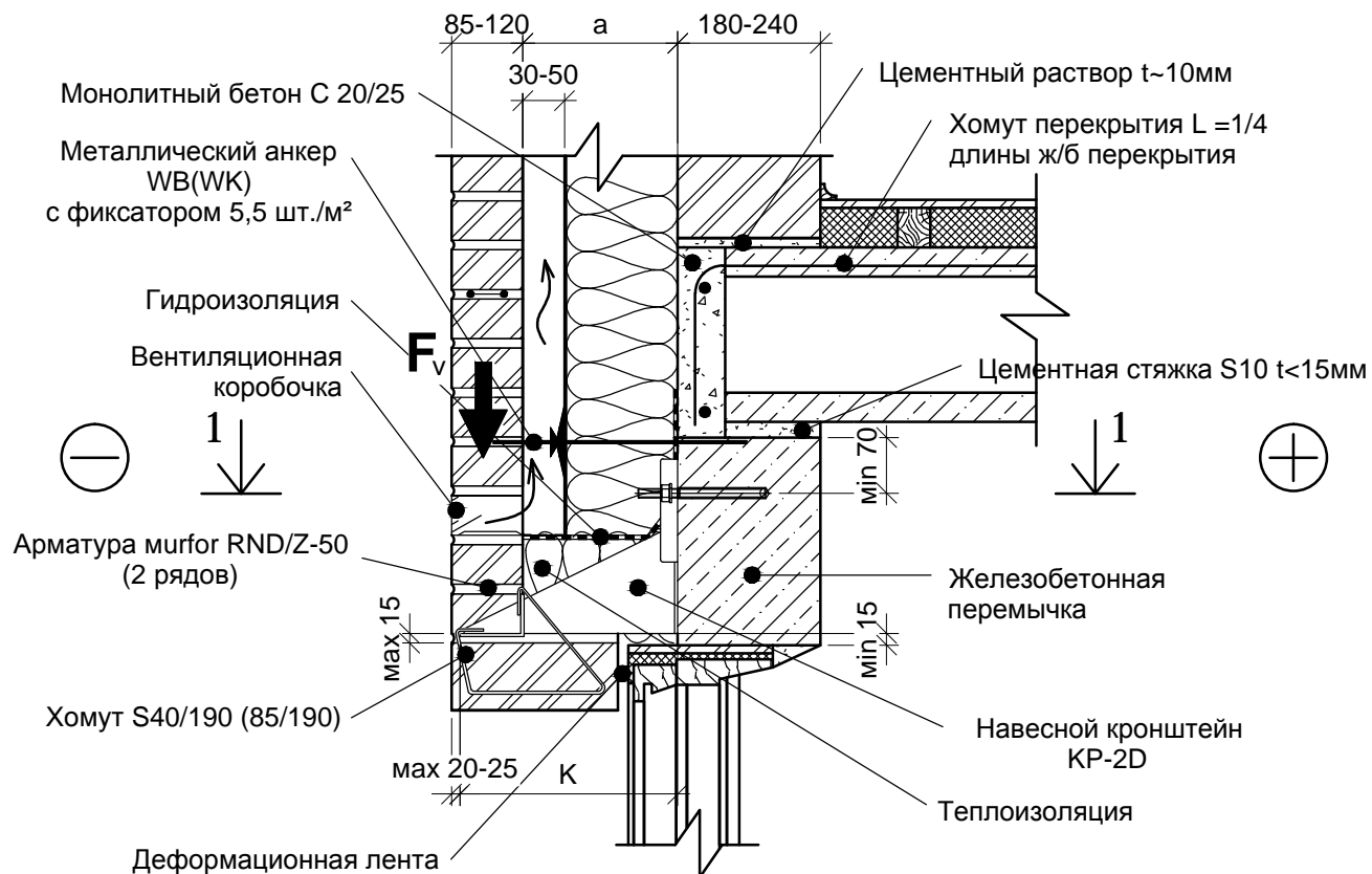
РАЗРЕЗ 1-1
