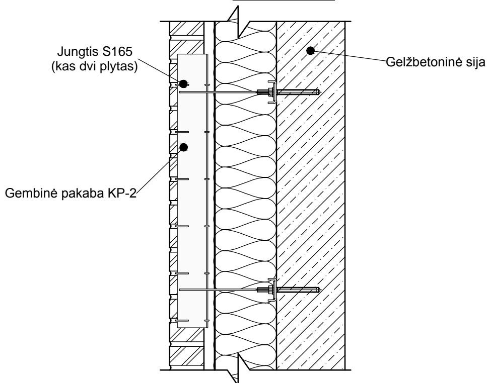
PJŪVIS 1-1
