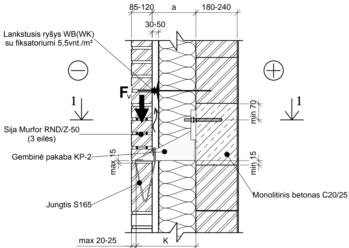
PJŪVIS 1-1
