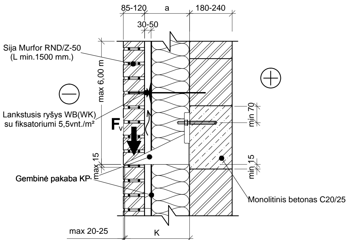
PJŪVIS 1-1
