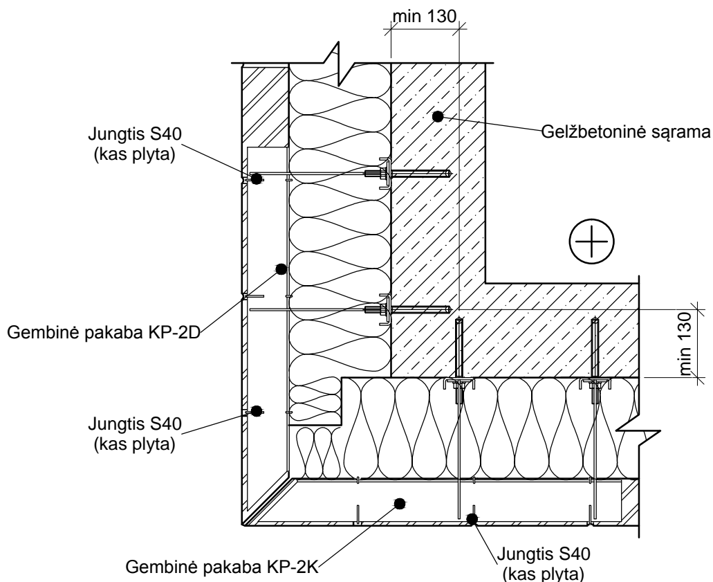
PJŪVIS 1-1
