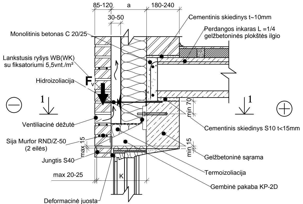
PJŪVIS 1-1
