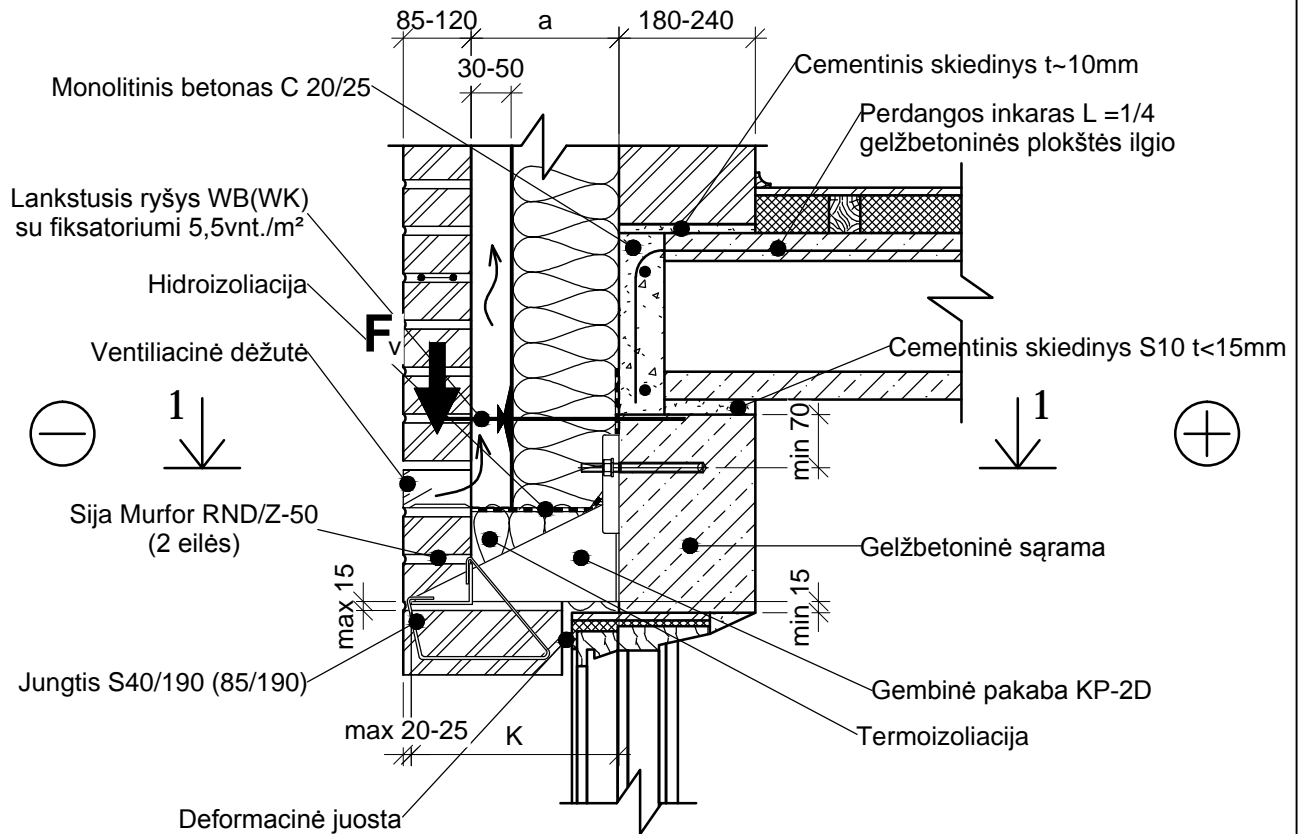
PJŪVIS 1-1
