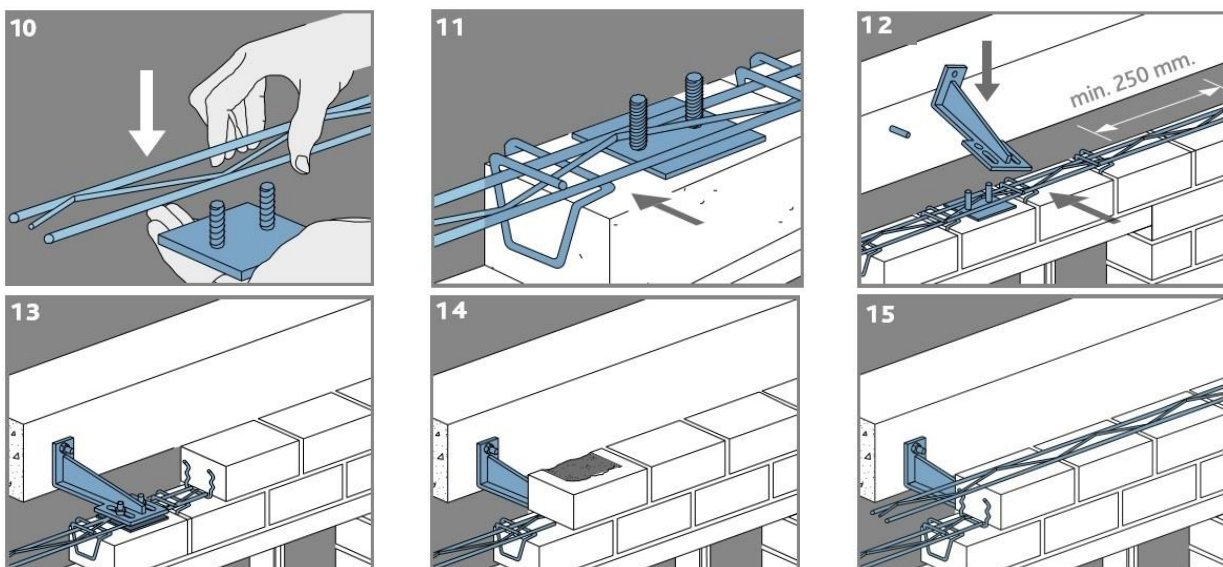
Показан монтаж кронштейна при горизонтальной кладке. Монтаж кронштейна аналогичен при всех типах кладки.
