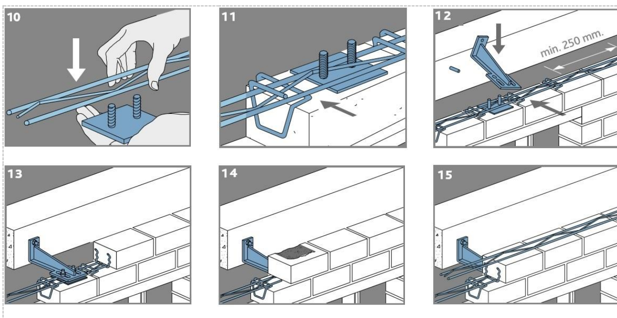
Parodytas horizontalaus dėjimo gembinės pakabos montavimas. Gembės montavimas visiems dėjimo būdams yra vienodas.
