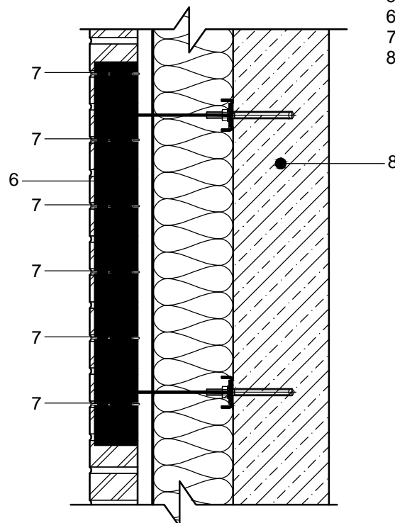
PLANAS pagal 1-1
