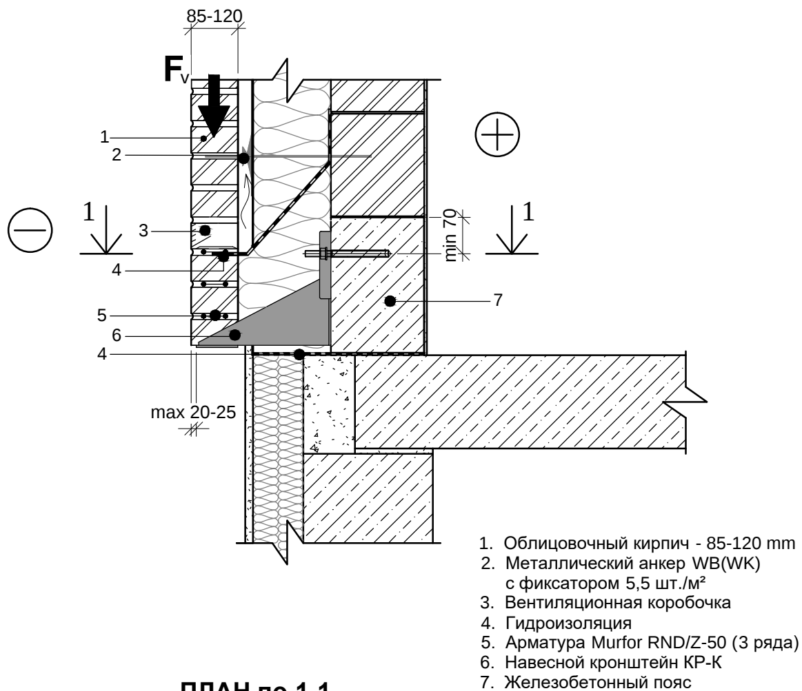
ПЛАН по 1-1
