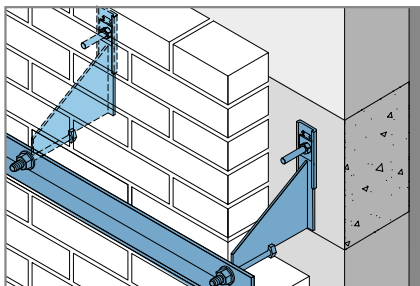
Кронштейн для присоединения конструкций
