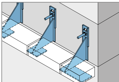
Правый и левый конечные кронштейны
