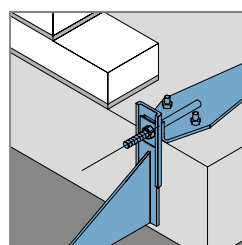
Крепление кронштейна к плите с помощью анкера PT-T2. В дальнейшем анкер закладывается стеновой конструкцией
