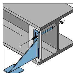
Крепление кронштейна
