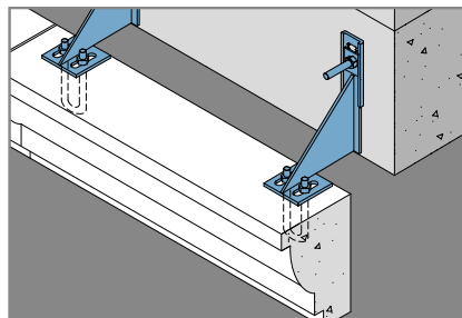
Вариант применения с навесными элементами заводского изготовления
