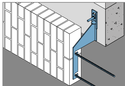
Кронштейн для крепления вертикальной кладки. Изготавливается индивидуально под формат кирпича.
