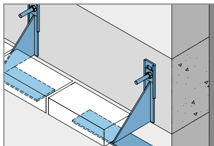
Рядовой кронштейн с удлиненной полкой
