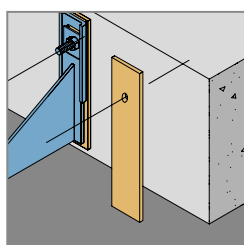
Для снижения теплотерерь между кронштейном и железобетонной конструкцией располагают термоизоляционную прокладку TS
