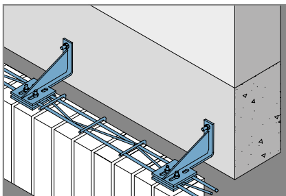
Рядовой кронштейн для кирпичных перемычек
