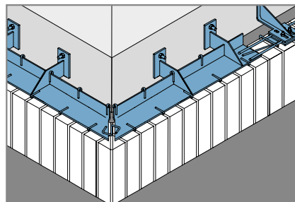
Правый и левый угловые кронштейны для перемычек
