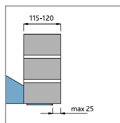
Допустимая величина свеса
