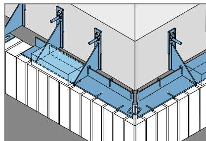
Правый и левый угловые кронштейны
