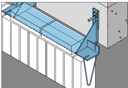
Рядовой двойной кронштейн с навешиванием нижнего ряда кладки
