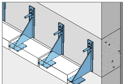
Рядовой кронштейн
